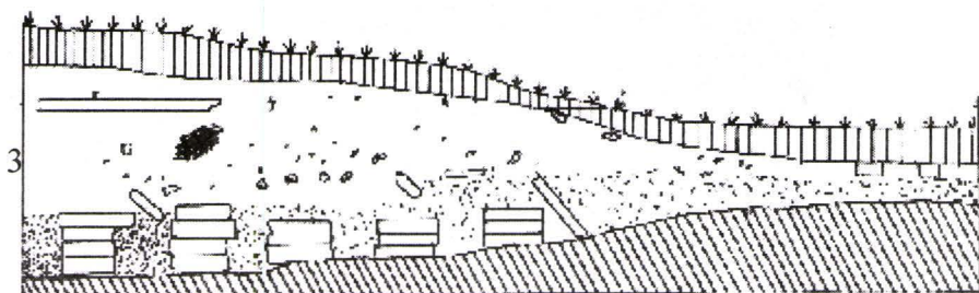
BUMBEȘTI JIU „VÂRTOP” - CAMPANIA 2002 - PROFILUL PERETEII DE SUD C 1 + C 2 / 2002 - sc.1/20
