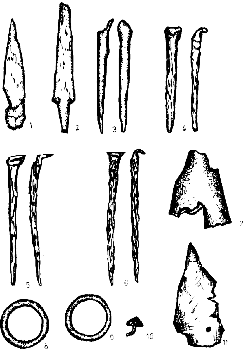
PI. X. OBIECTE ROMANE DIN METAL DESCOPERITE LA CIOCADIA „Codrișoare” (2002) Scara 1/2 .- 1,2 fragmente cuțit fier; 3,4,5,6 piroane din fier; 7,11 fragmente coif fier; 8,9 verigi bronz; 10 țintă fier.
